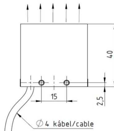
Oldalnézet/Side view
