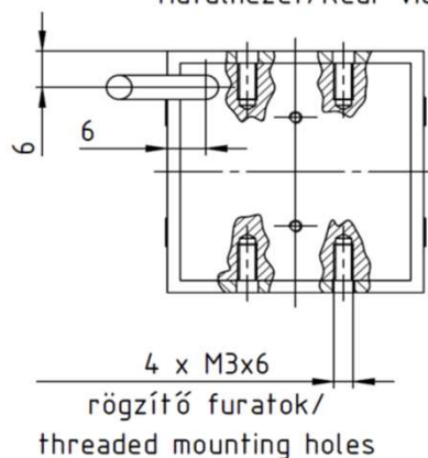
Hátulnézet/Rear view
