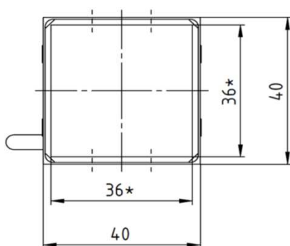
Előlnézet/Front view
